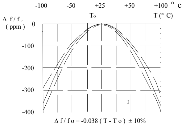
湖南海天电子有限公司 HUNAN HORIZON ELECTRONICS CO.,LTD. 频率温度曲线图 Frequency Temperature Curve
